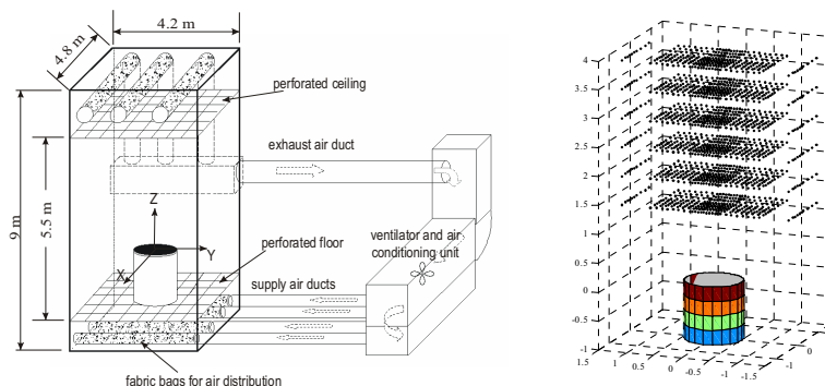
Kuva 5.2. Mittausjärjestelyt.
