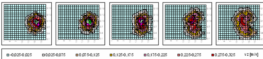
Kuva 5.6. Jettihäiriön vaikutus pluumin. Nopeus vaakatasolla 3 m korkeudella lämpötehoalla 594 W. Häiriönopeudet vasemmalta 0 m/s, 0,25 m/s, 0,5 m/s, 0,75 m/s ja 1,0 m/s.
