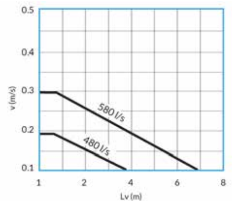
Deco.UH-5020
