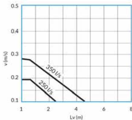
Deco.UH-4020
